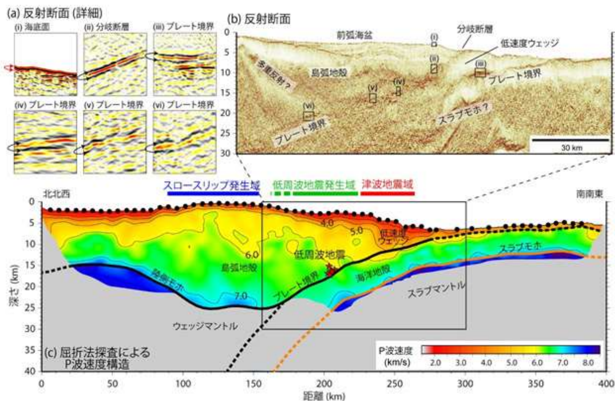
図3 琉球海溝南部の構造。(a, b)反射法探査によるイメージ。プレート境界と分岐断層が明瞭にイメージングされている。この分岐断層と低速度ウェッジの位置は先行研究で推定されている1771年八重山地震による津波発生域と重複し
