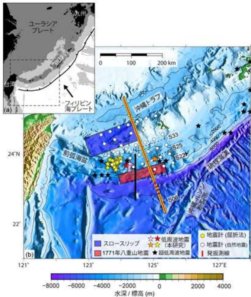
図1 観測点配置と観測した低周波地震の分布。(a)琉球海溝の広域図。(b)調査海域図。発振側線(赤線)上に海底地震計(黄色丸印)を設置し、エアガン発振(容量7800立方インチ)によって屈折法データを取得するとともに、同測線上で6km長のストリーマケーブル(チャンネル数444)を曳航し、反射法データを取得した。また、石垣島・西表島周辺に設置した海底地震計(白色丸印)および陸上地震計による3カ月間の自然地震観測も実施した。色付き星印は本観測で決定した低周波地震の震央位置。観測した73個の低周波地震は4つのグループ(ピンク・オレンジ・赤・黄色に対応)から成る。黒星は過去に観測された超低周波地震の震央位置。赤四角は先行研究で推定されている1771年八重山地震の震源域。青四角は過去観測されているスロースリップ発生域。
