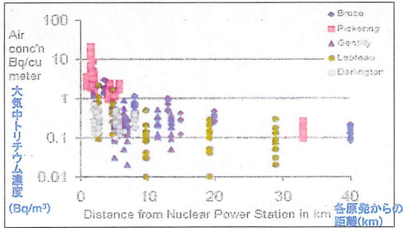
1985～1999年のカナダの5原発からの距離と年平均の大気中トリチウム濃度。
