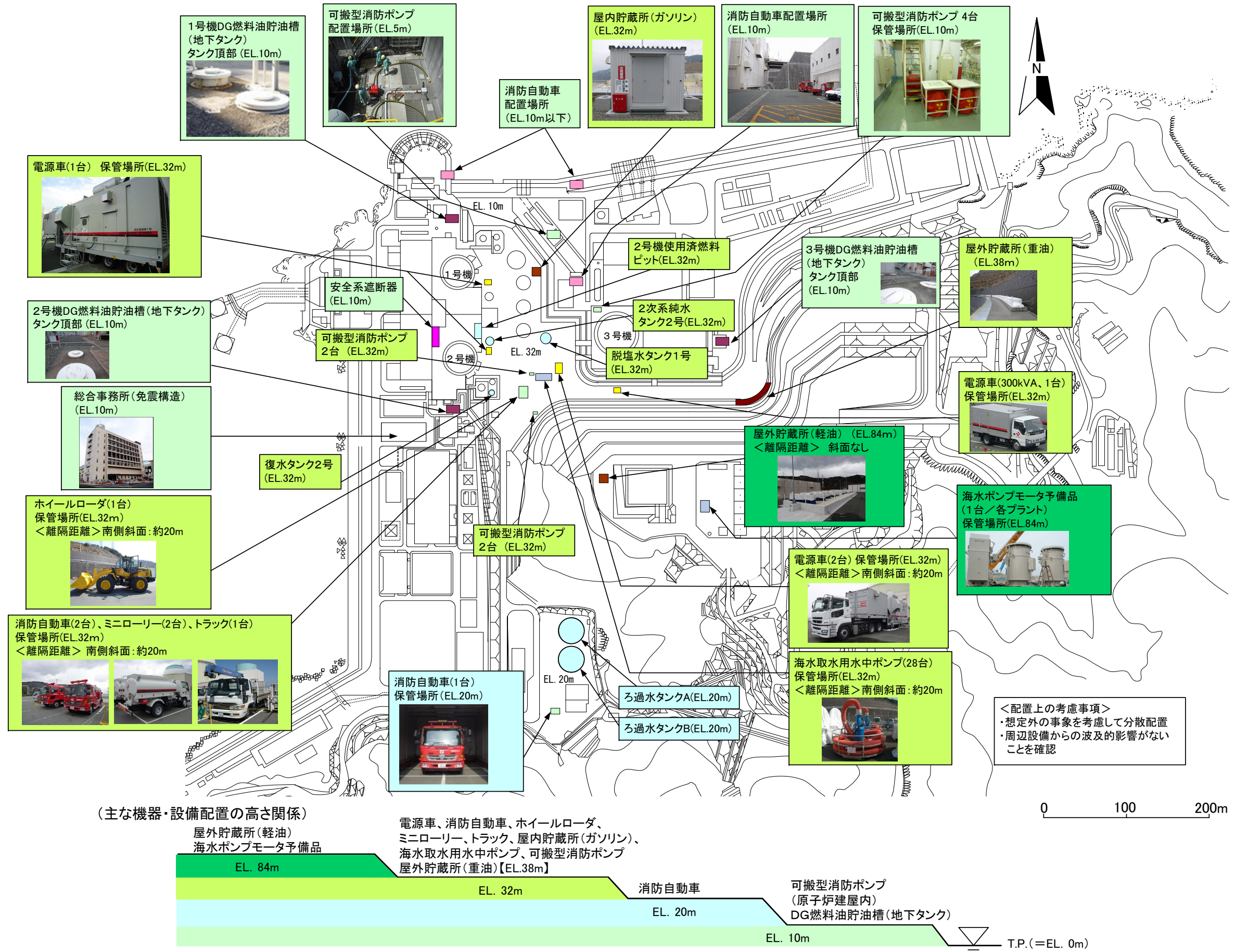
緊急安全対策に係る資機材配置図
