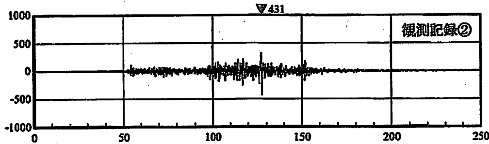
図2—上：Ss-L(水平方向) 川内原発「設置変更許可申請書」第7.5.7.11図より転載。 下：福島第一6号機原子炉建屋基礎版上の加速度時刻歴波形(東西方向) 東京電力「福島原子力事故調査報告書(中間報告書，2011年12月2日)」添付3-2 図1-6より転載。
