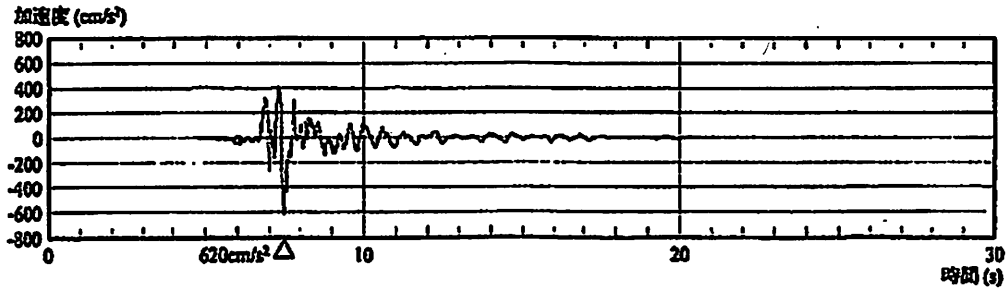
図1—上：Ss-1(水平方向)，下：Ss-2(水平方向) それぞれ，川内原発「設置変更許可申請書」第7.5.6.58図，第7.5.6.59図より転載。
