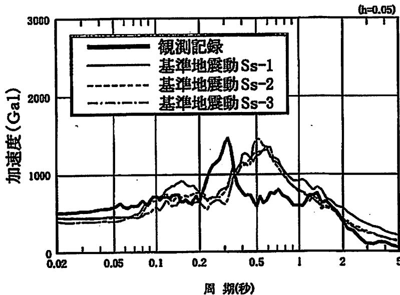
図4—福島第一3号機原子炉建屋基礎版上の 応答スペクトル(東西方向) 東京電力「福島原子力事故調査報告書(中間 報告書, 2011年12月2日)」添付3-2 図 2-3より転載。
