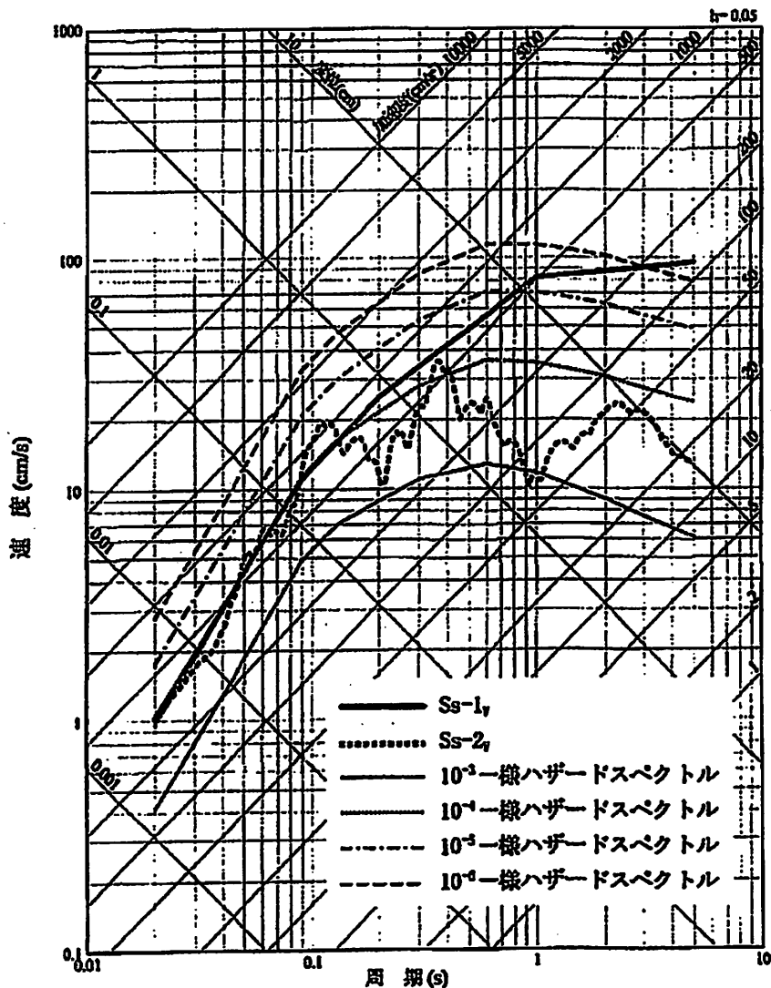
図3—基本地震動の応答スペクトル及び日本原子力学会(2007)の方法により算定した解放基盤表面における地震動の一概ハザード・スペクトルの比較(鉛直方向) 川内原発「設置変更許可申請書」第7.5.6.61図より転載。
