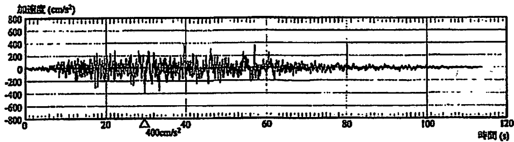
図1—上：Ss-1(水平方向)，下：Ss-2(水平方向) それぞれ，川内原発「設置変更許可申請書」第7.5.6.58図，第7.5.6.59図より転載。
