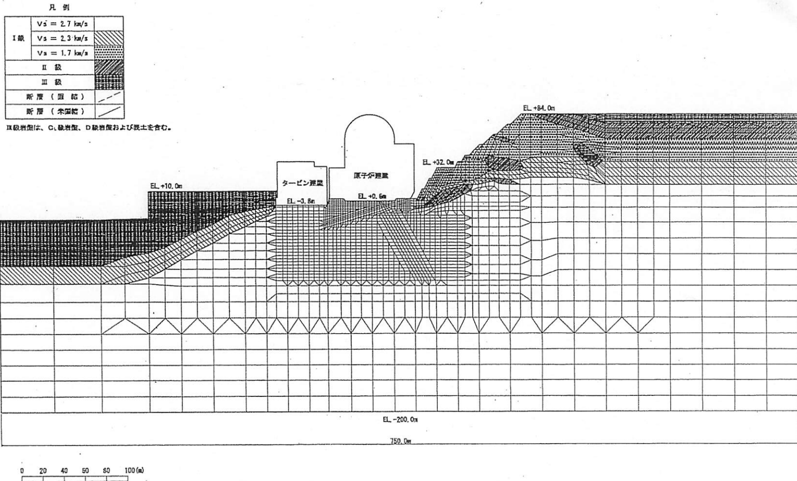
第 3.1-2 図 解析用要素分割図 (X-X' 断面)
