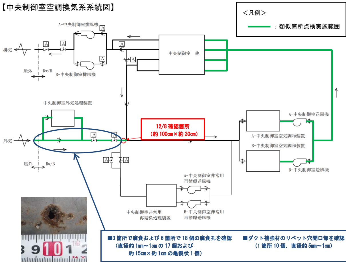
【中央制御室空調換気系ダクト配置イメージ図】
