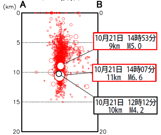
震央分布図の矩形内の断面図
