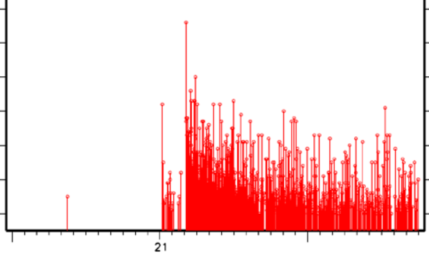
2016年10月21日0時～22日9時、 M \geq 1.0
