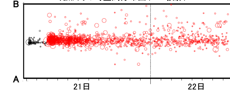
矩形内の時空間分布図 (B-A投影)
