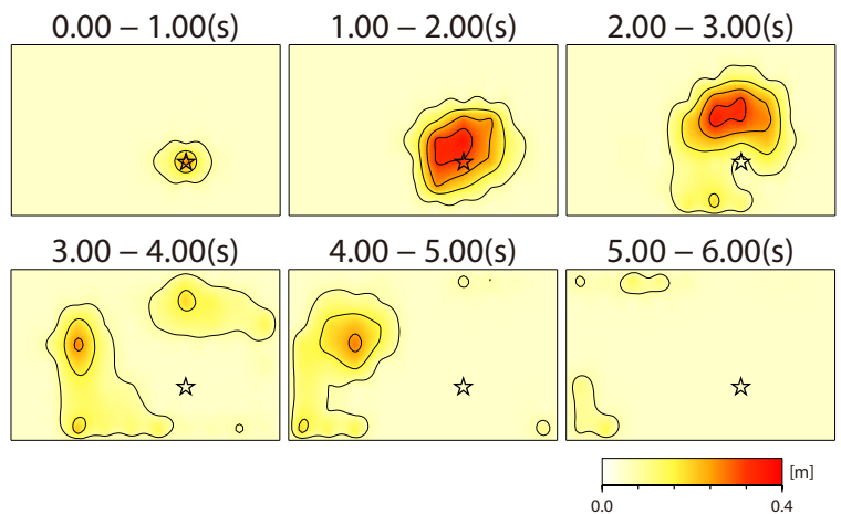
図4: 破壊の時間進展過程。1.0秒ごとのすべり分布を地表投影している。
