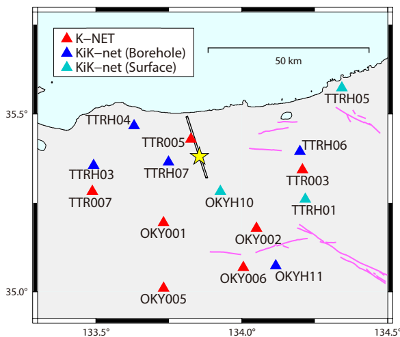
図1: 観測点の分布及び断層面の地表投影。星印は破壊開始点を示す。
