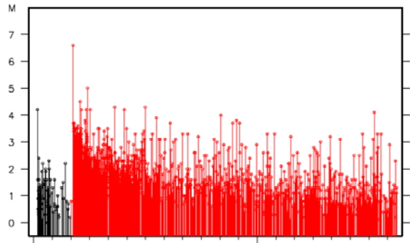
矩形内のMT図及び回数積算図
