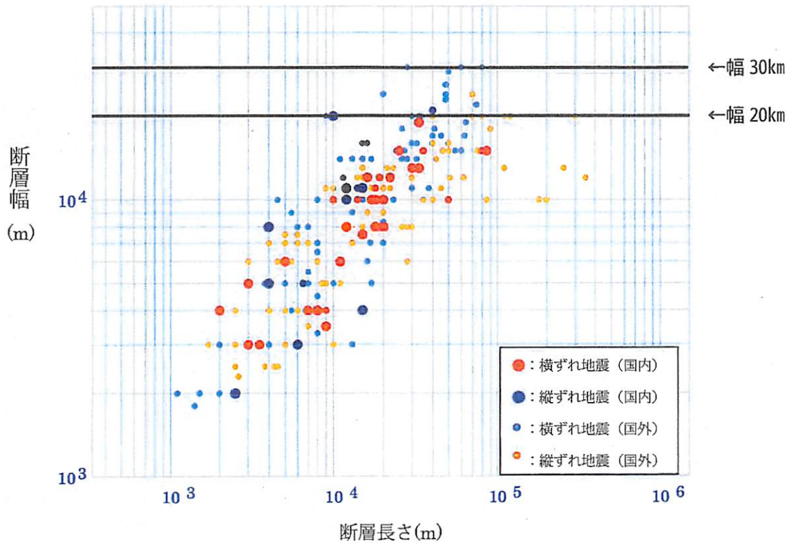
図 2.2.1 断層の長さと断層幅の関係
