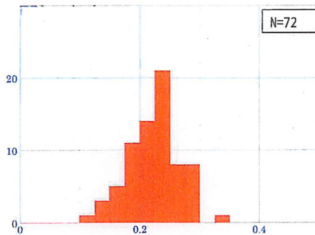
図 2.4.3 アスペリティ面積率の度数
