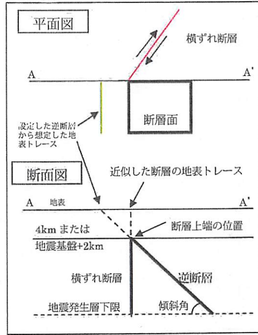
a) 逆断層のみまたは横ずれ断層のみでモデル化した場合 b) 横ずれ断層と逆断層からなる断層帯の場合
