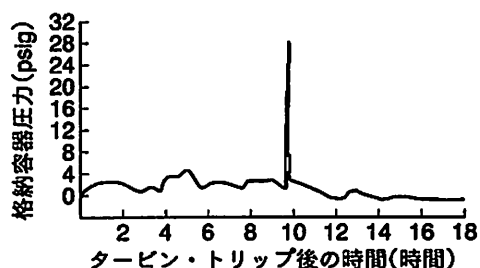
図7—米国スリーマイル島原子炉事故時の格納容器内圧力変化
