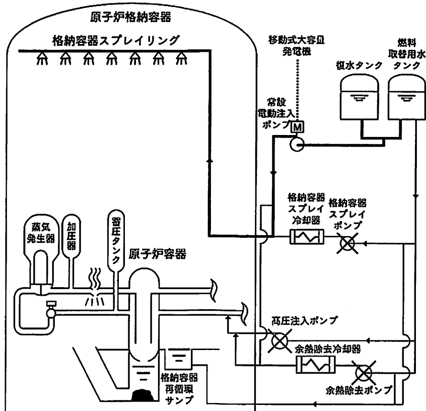
図2—図1の事故対策シナリオに対応する設備構成の概要(玄海3・4号の設置変更許可申請書掲載図より主要部抜粋)
