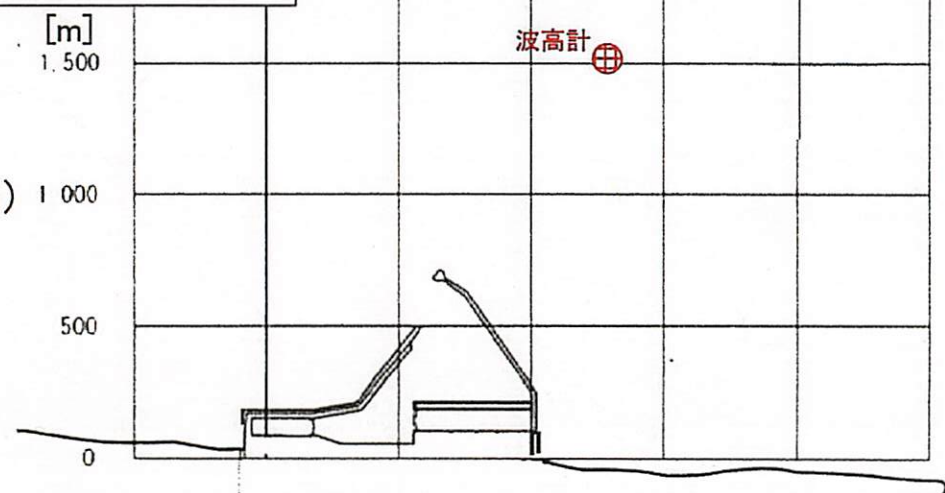
福島第一原子力発電所における波高計の設置位置図
